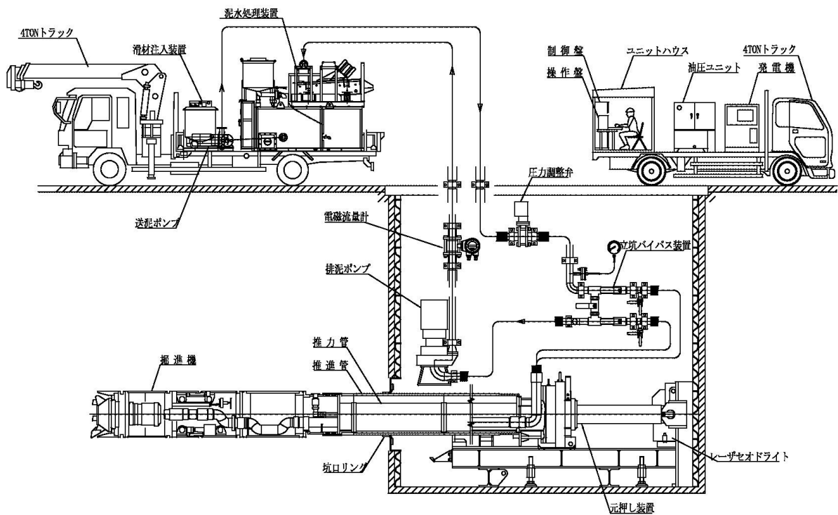
図 2-1 アンクルモールV工法系統図
